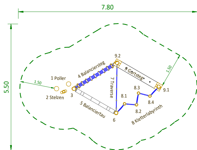
Draufsicht
