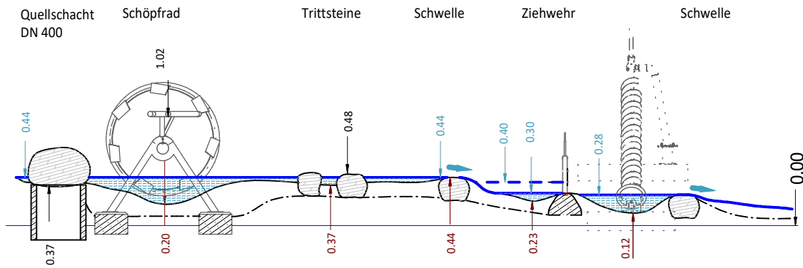
Schöpfrad
